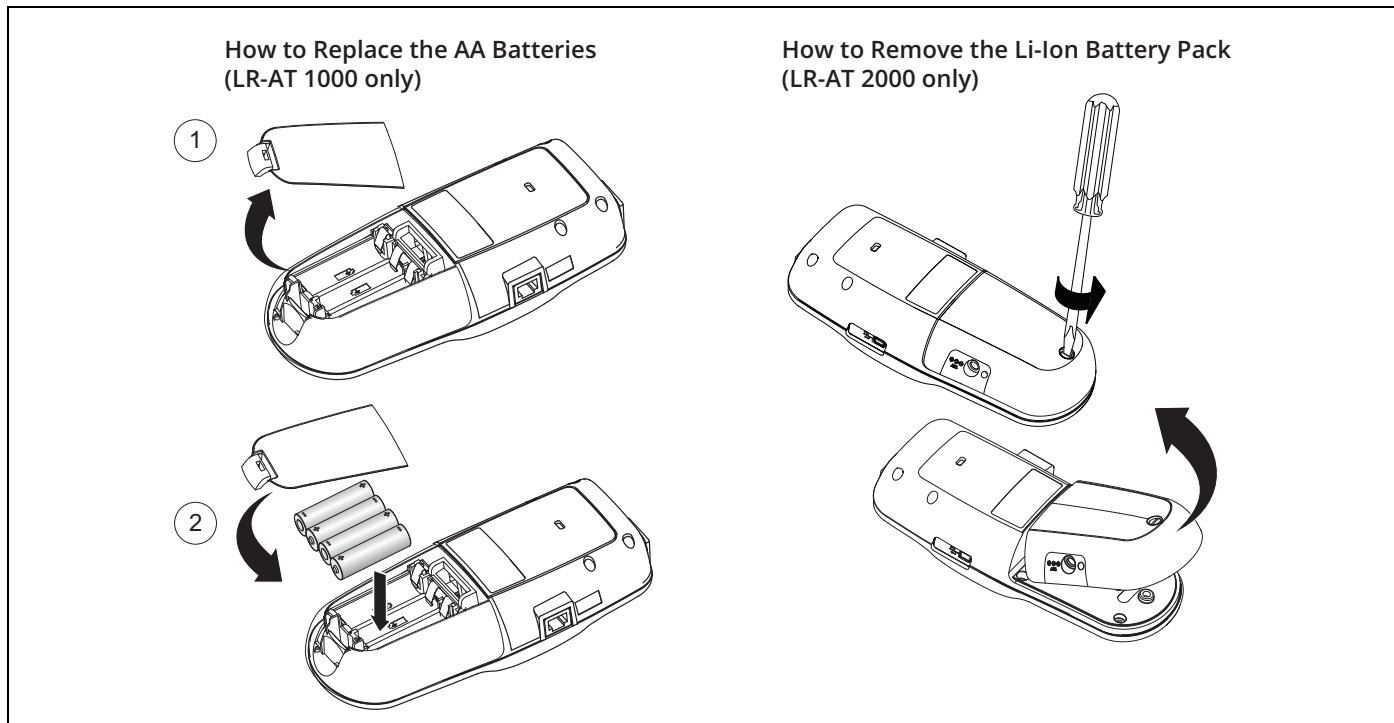
Figura 2. Como remover/substituir as baterias
